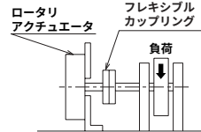
図2 (ラジアル荷重)
